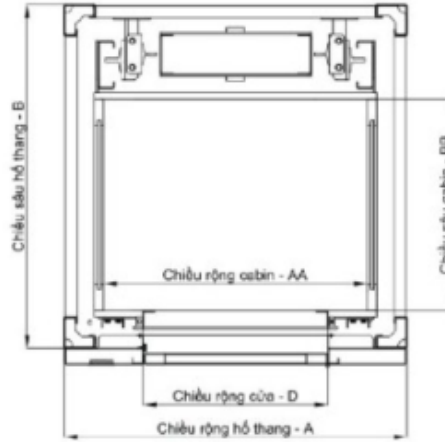
MẶT CẮT NGANG HỒ THANG – ĐỐI TRỌNG MẶT LƯNG
