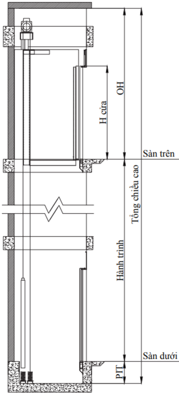
MẶT CẮT DỌC HỒ THANG
