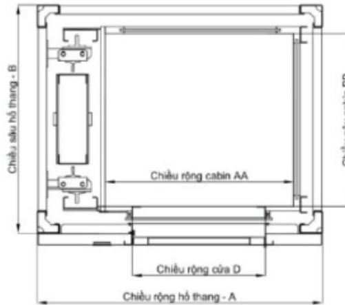
MẶT CẮT NGANG HỒ THANG – ĐỐI TRỌNG MẶT HÔNG
